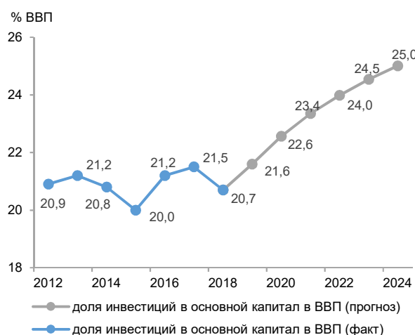
Рис. 11. К 2024 году доля инвестиций в основной капитал в ВВП достигнет 25 %
