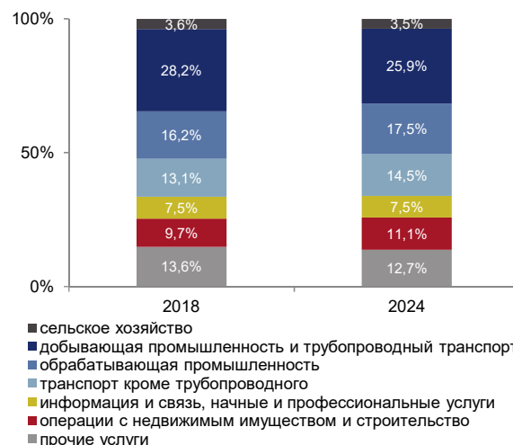
Рис. 12. В отраслевой структуре инвестиций произойдут сдвиги
