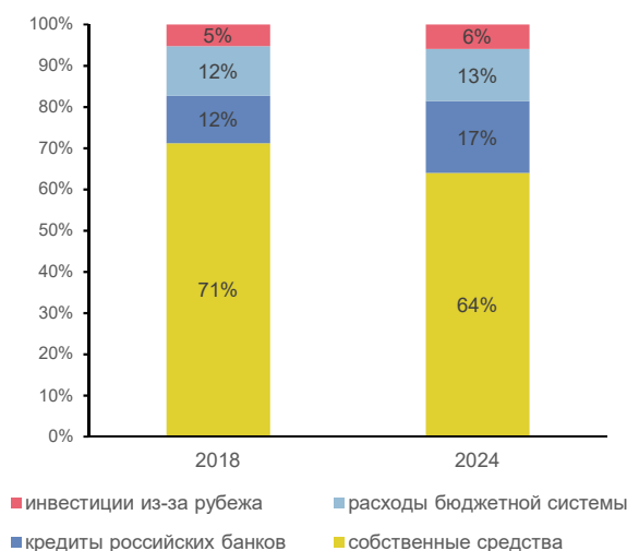
Рис. 13. Структура инвестиций в основной капитал по источникам финансирования
