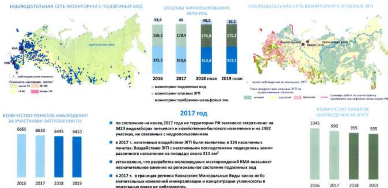
Рис. 4. Мониторинг состояния геологической среды
