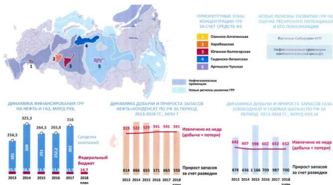
Рис. 5. Приоритетные направления по воспроизводству минерально-сырьевой базы УВС
