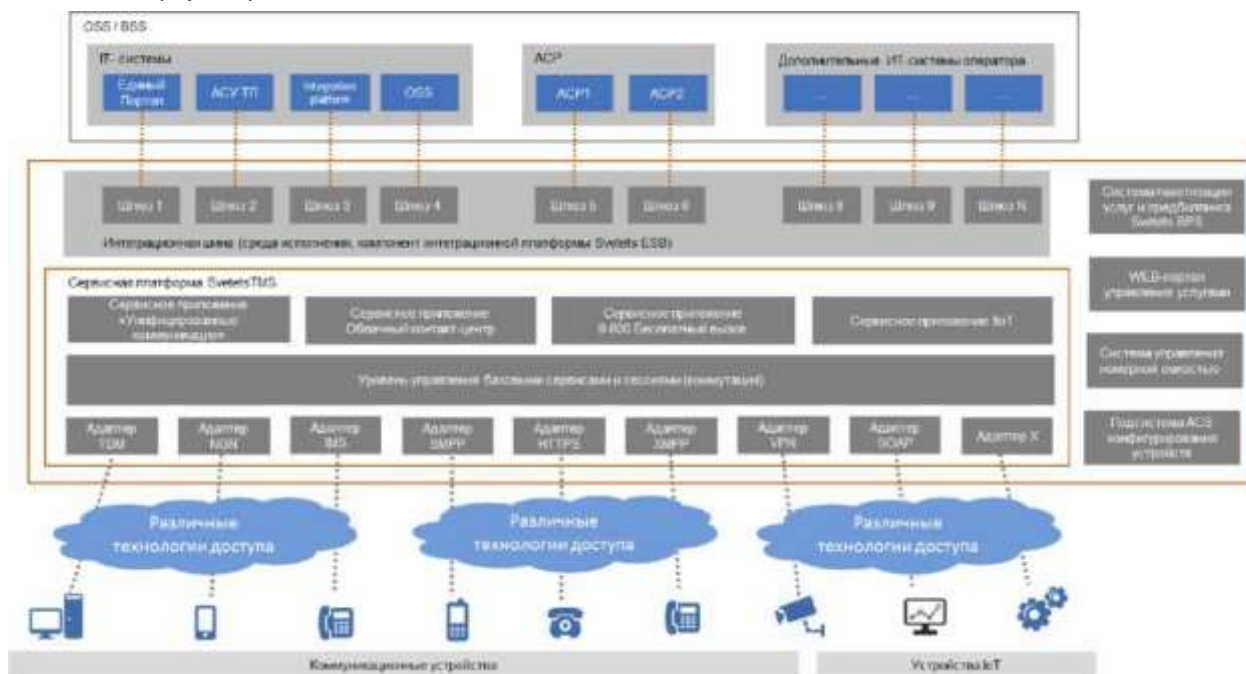
Рис. 1. Архитектура Платформы универсальных коммуникаций
