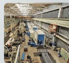
Габаритный порталный VMB 3200x4000
